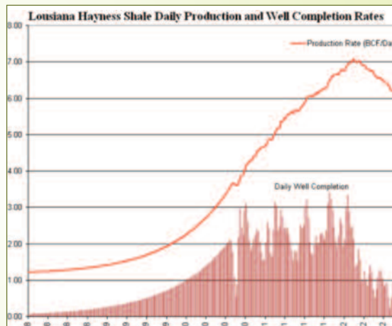
Fig.2. Een van de grootste schalie gas winningen (Louisiana Haynes Shale) heeft thans duidelijk een plafond bereikt
